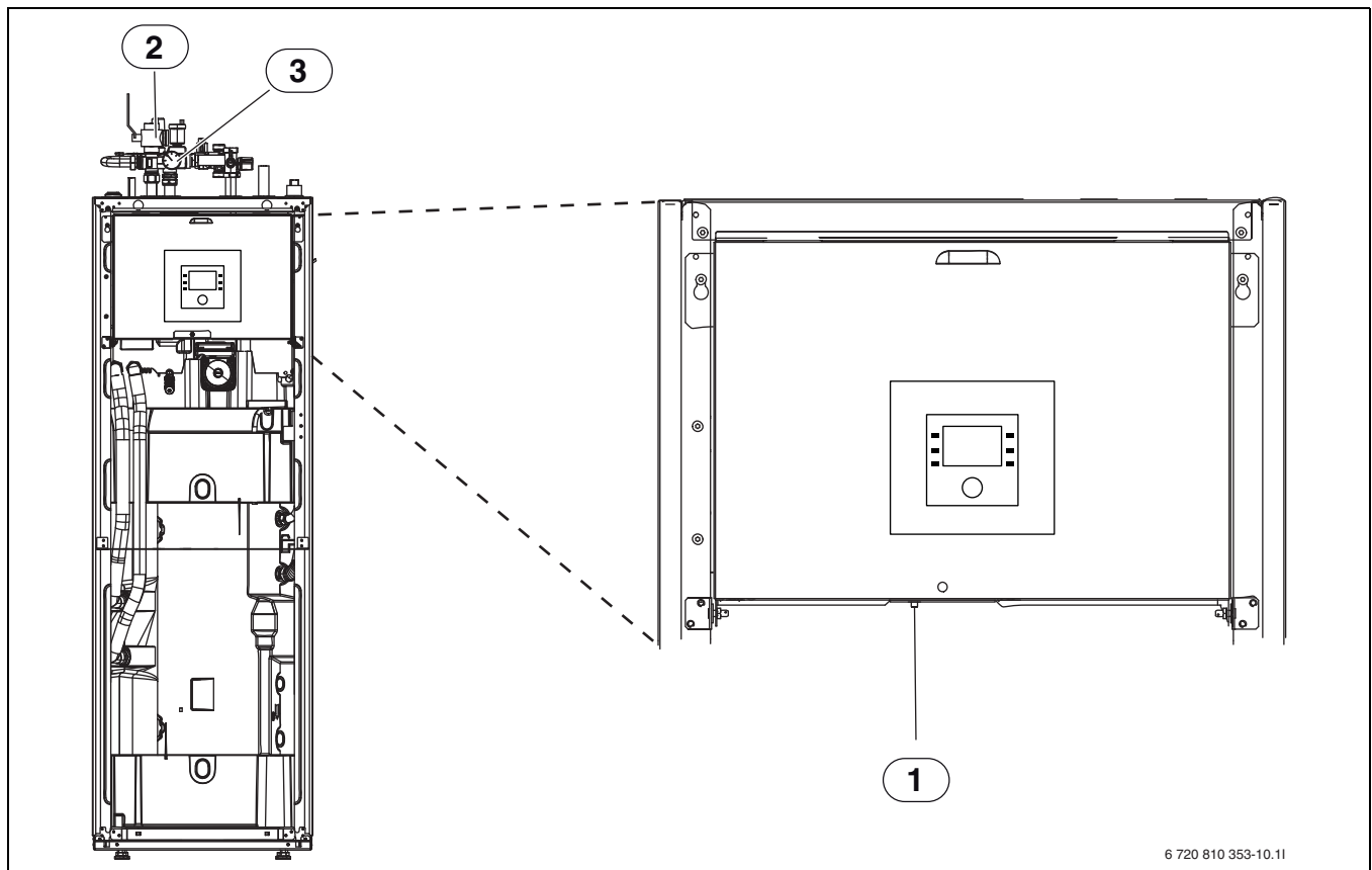
7. ábra AWMS/AWMS szolár beltéri egység
