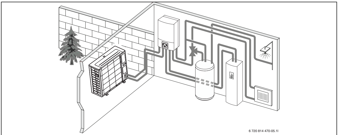
3. ábra Hőszivattyú kültéri egység, AWBS beltéri egység elektromos rásegítő fűtő, külső melegvíz-tároló és külső rásegítő fűtő nélkül
