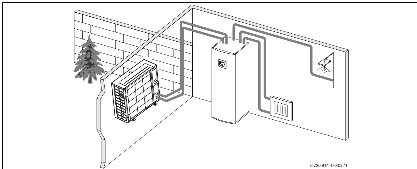
1. ábra Hőszivattyú kültéri egység, AWMS/AWMSS beltéri egység beépített melegvíz-tárolóval és elektromos rásegítő fűtővel
