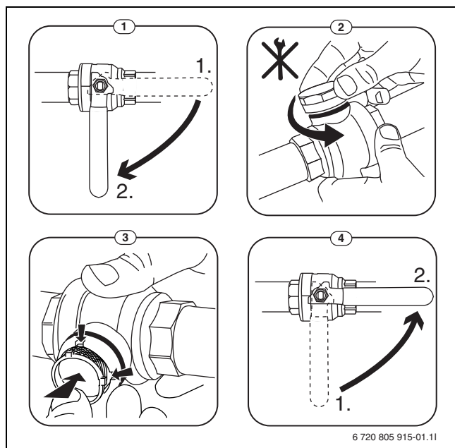
5. ábra Biztosító gyűrű nélküli szűrőváltás
