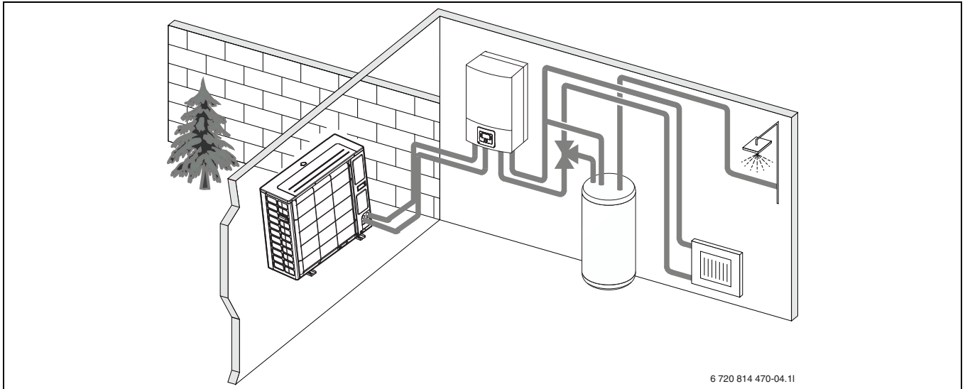
2. ábra Hőszivattyú kültéri egység, AWES beltéri egység elektromos rásegítő fűtővel, külső melegvíz-tárolóval
